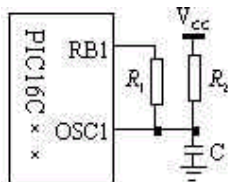
图 1 提高工作频率的方法
